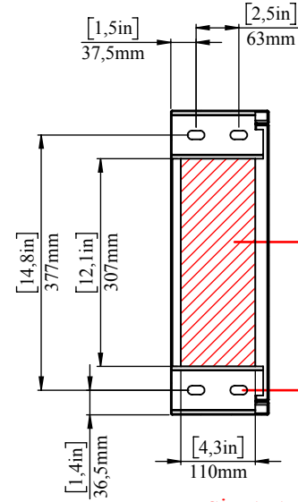
KESİT A-A
